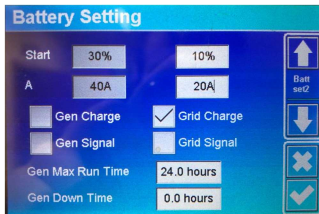
Obrázek 4: Nastavení baterie 2
