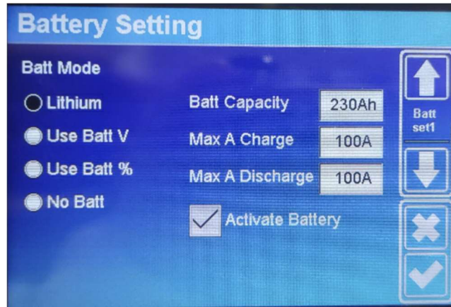
Obrázek 3: Nastavení baterie 1
